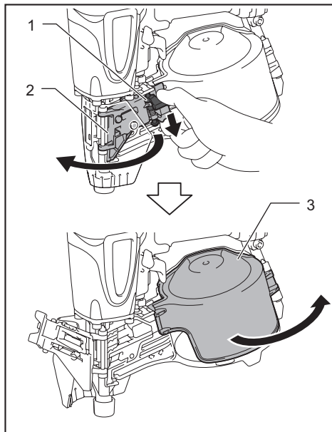
► 1. Palanca del seguro 2. Compuerta 3. Tapa del cartucho
